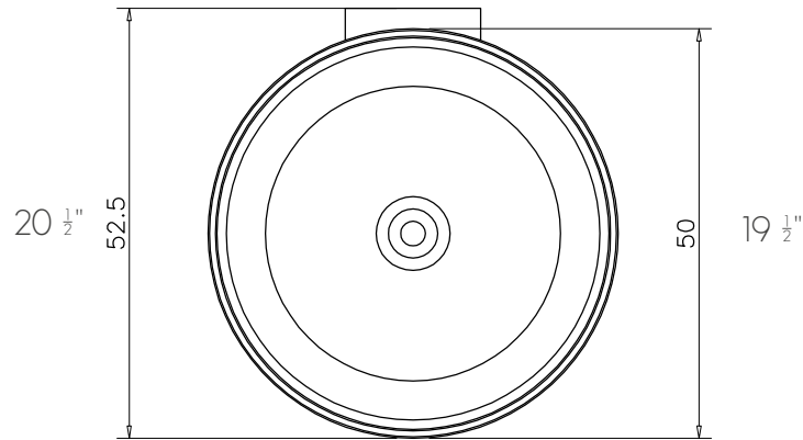
SUPERIOR / TOP
