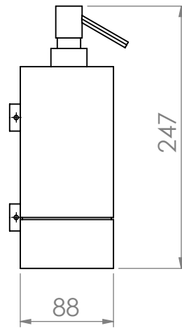
FRONTAL
