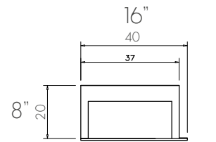
SUPERIOR / TOP
