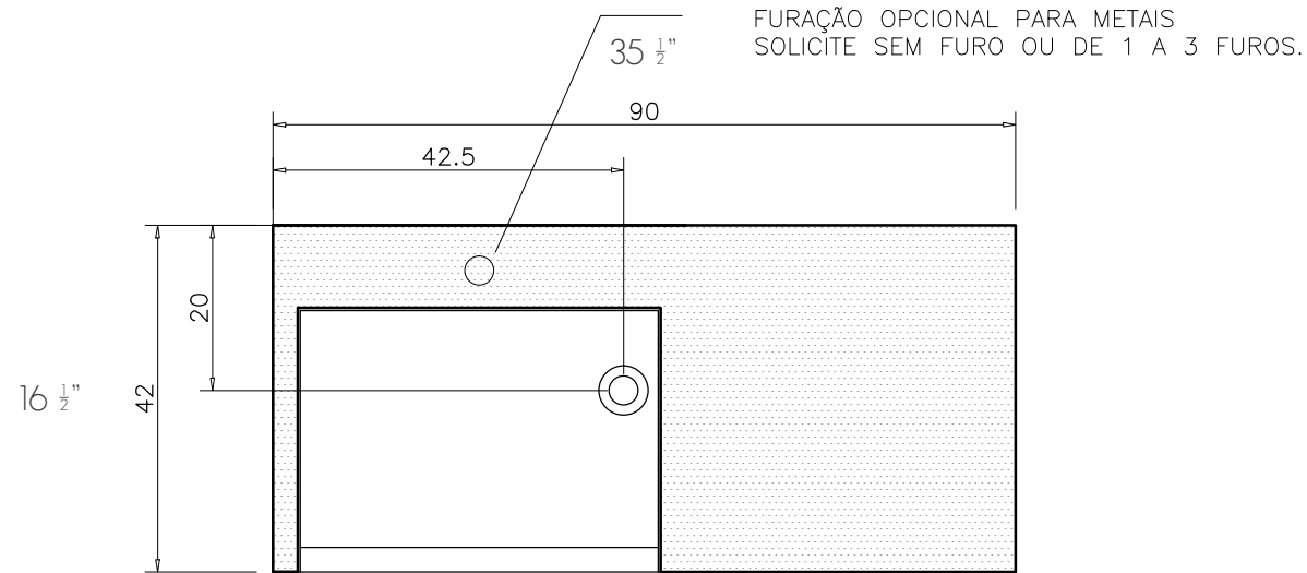
SUPERIOR / TOP
